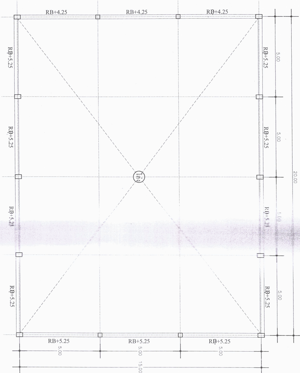
แปลนโครงสร้างคานรับโครงสร้างคาน Scale 1:100
